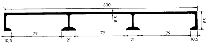
AS31118 Δ 3,31 kg/m code 530209 6,025 m
