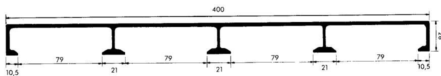
AS31118 Δ 3,31 kg/m code 530209 6,025 m
